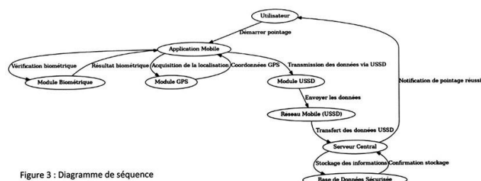
Figure 3 : Diagramme de séquence
