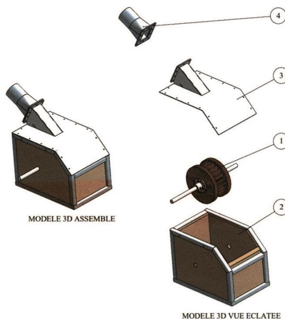
Figure : Vue éclatée de la turbine crossflow avec des essences spécifiques de bois
