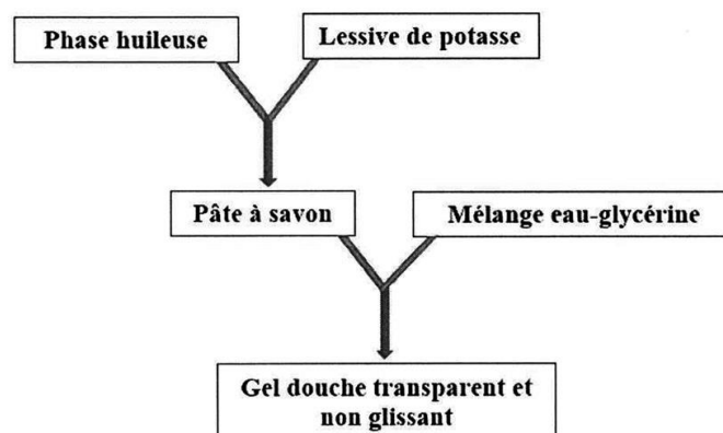
Figure 1 : synoptique de la fabrication du gel douche
